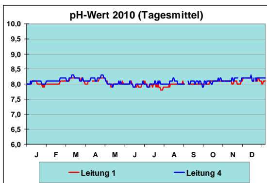
Abb. 1.3.3: pH-Wert, Jahresgang 2010
