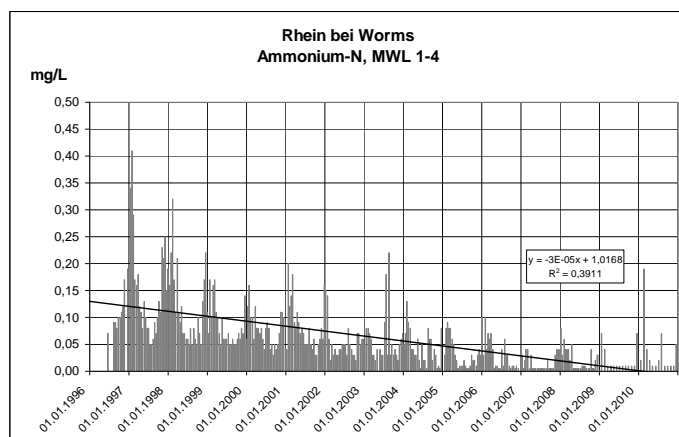
Abb. 1.3.5: Ammonium-N 1996-2010
